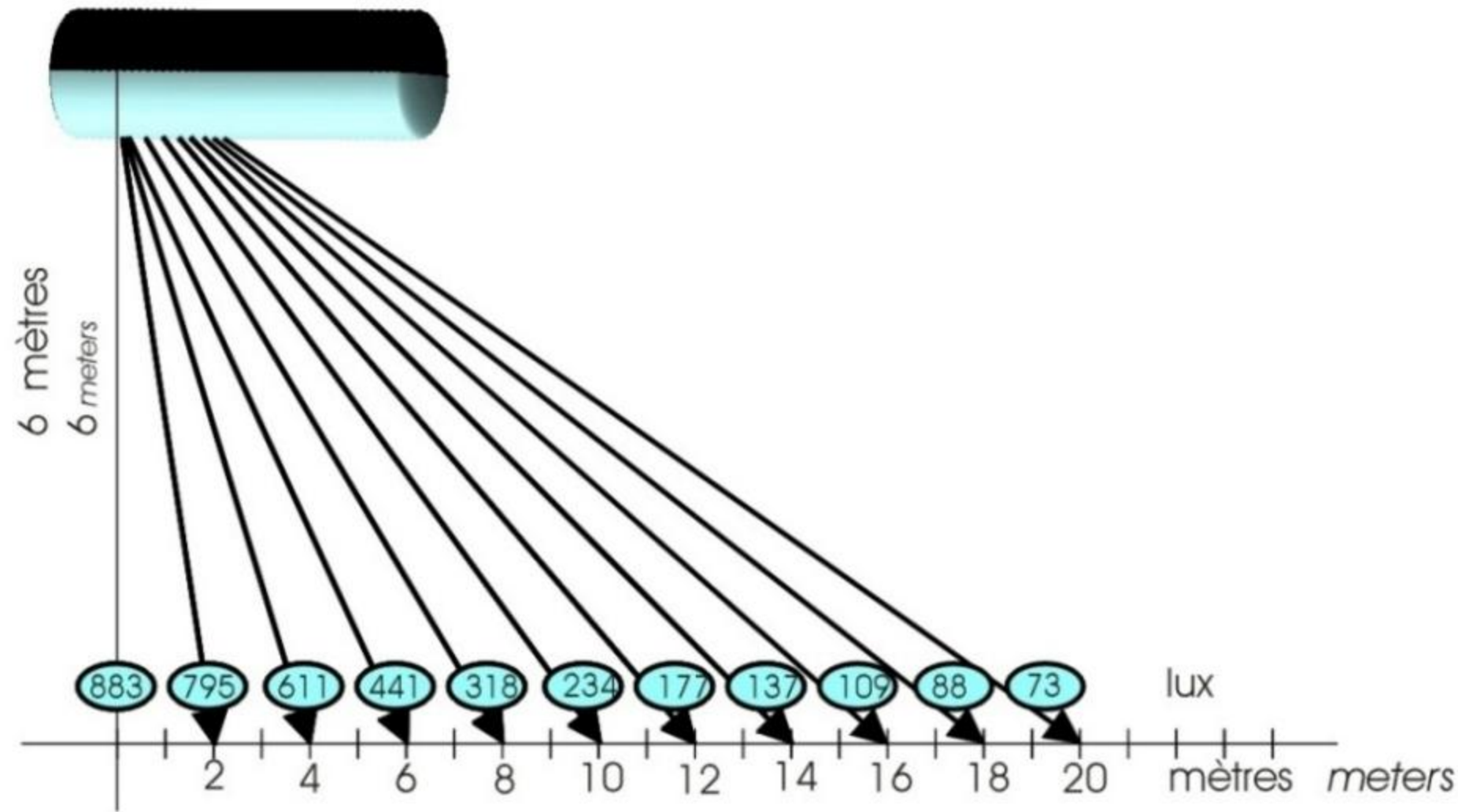
Flux lumineux du Tube 440 HH
