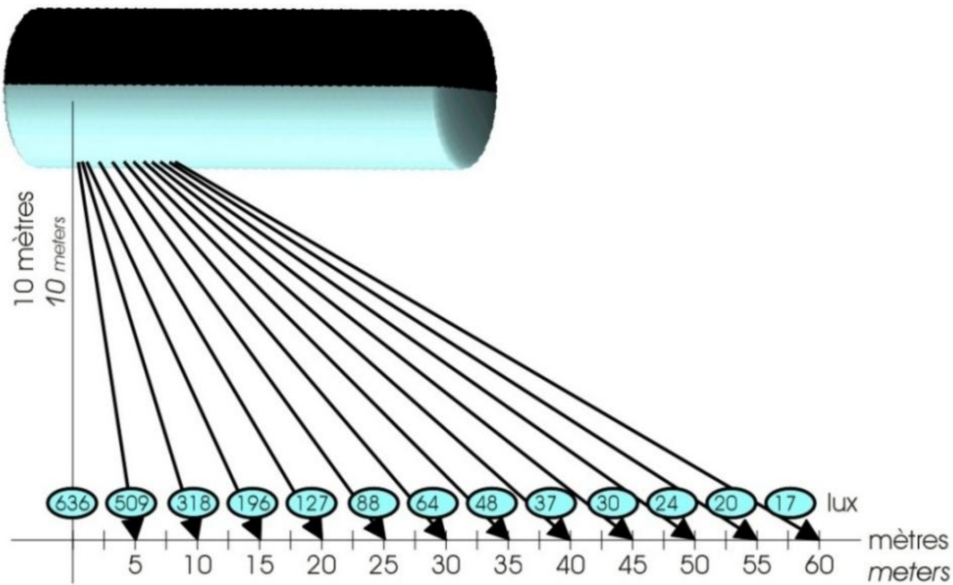
Flux lumineux du Tube 1280 HH
